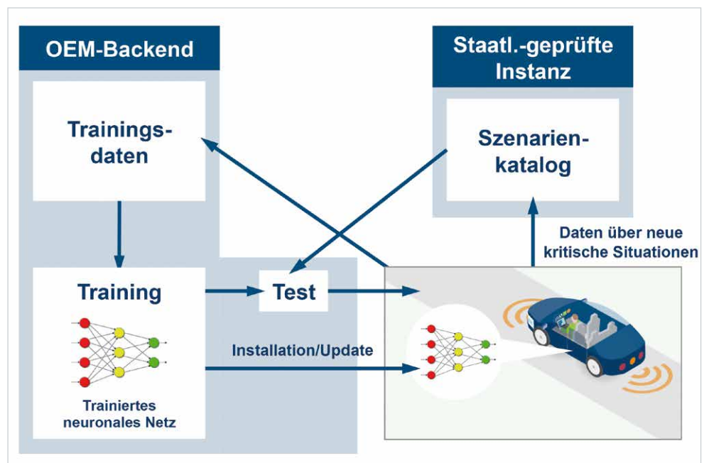
Abb. 3: Aufbau einer Wissensbasis zu kritischen Fahrfunktionen durch End-to-end Deep Learning (eigene Darstellung)
